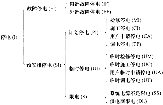
图 1 停电性质分类
